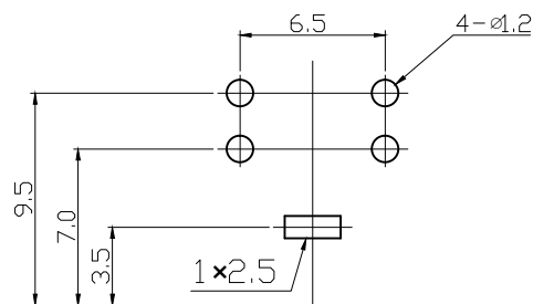
PCB板安装孔图
